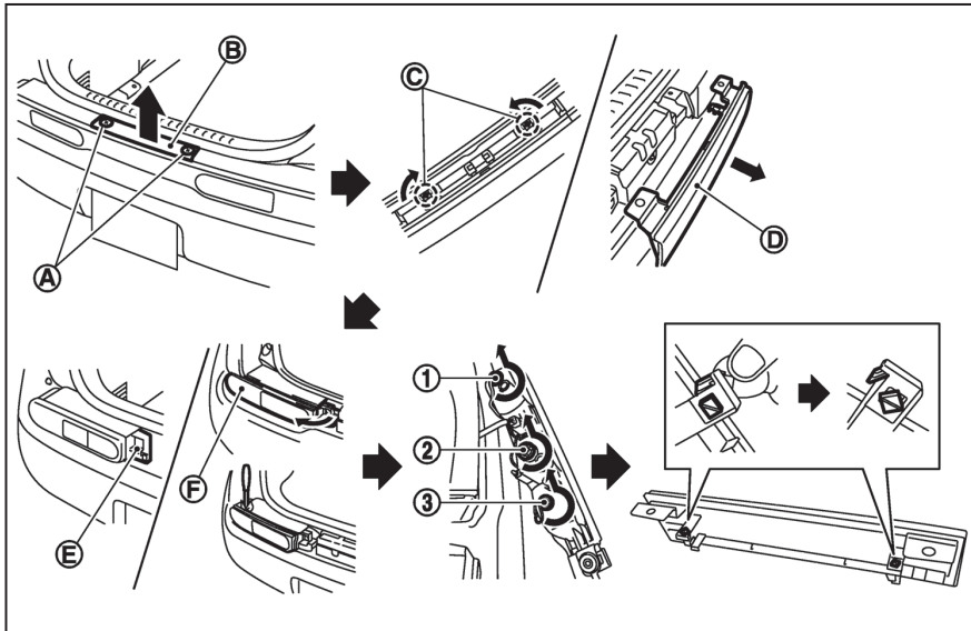
후방 콤비등
