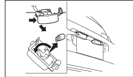
번호판등
