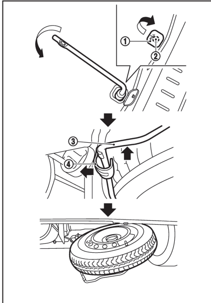
스페어 타이어
