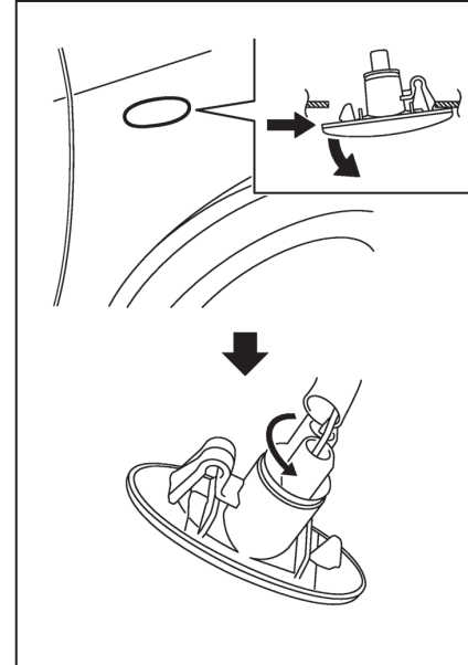
측면 방향지시등
