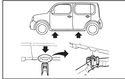
잭 받침부
