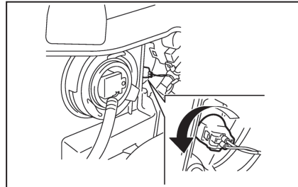
차폭등
